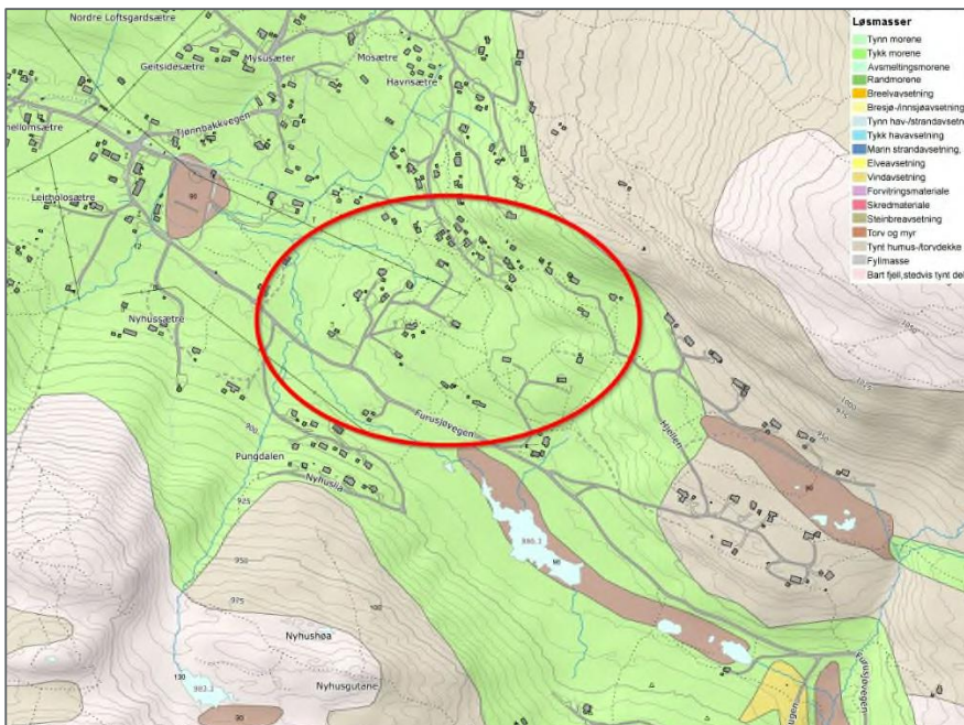
Figur 5. Løsmassekart (NGU, 2021) for området med tegnforklaring. Planområdets omtrentlige plassering i kartutsnitt er markert med rødt omriss.
