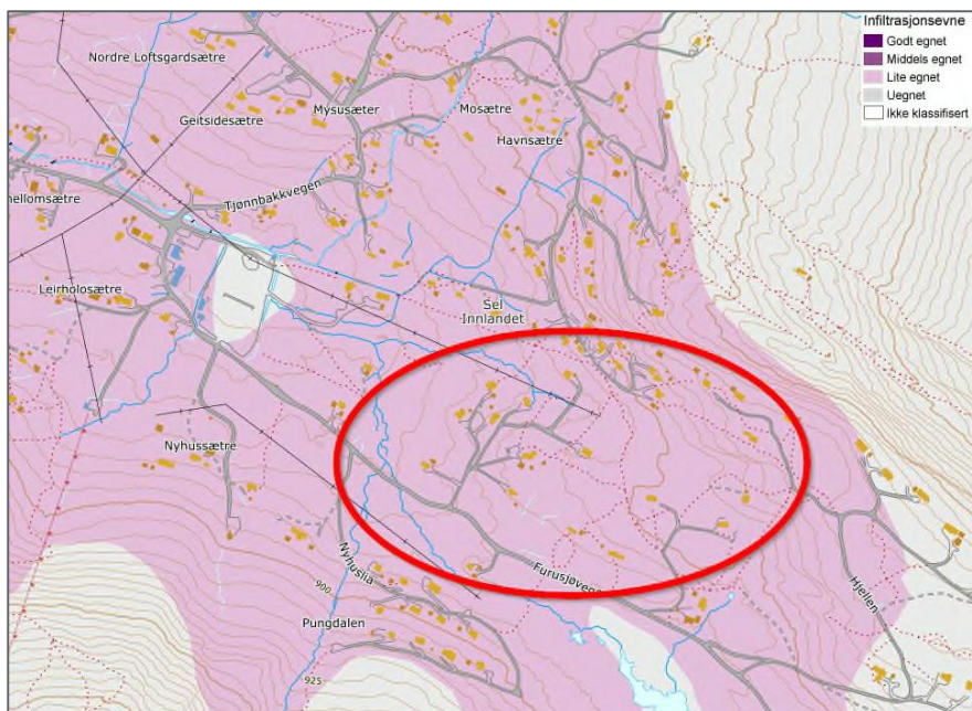
Figur 6. Infiltrasjonsevne (NGU, 2021) for området med ca. Planområdets omtrentlige plassering i kartutsnitt er markert med rødt omriss.
