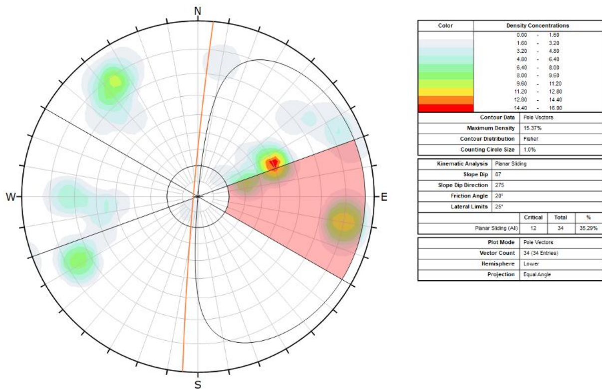
Figur 10: Analyse for planutglidning for skjæring mellom profil 2300-2900.
