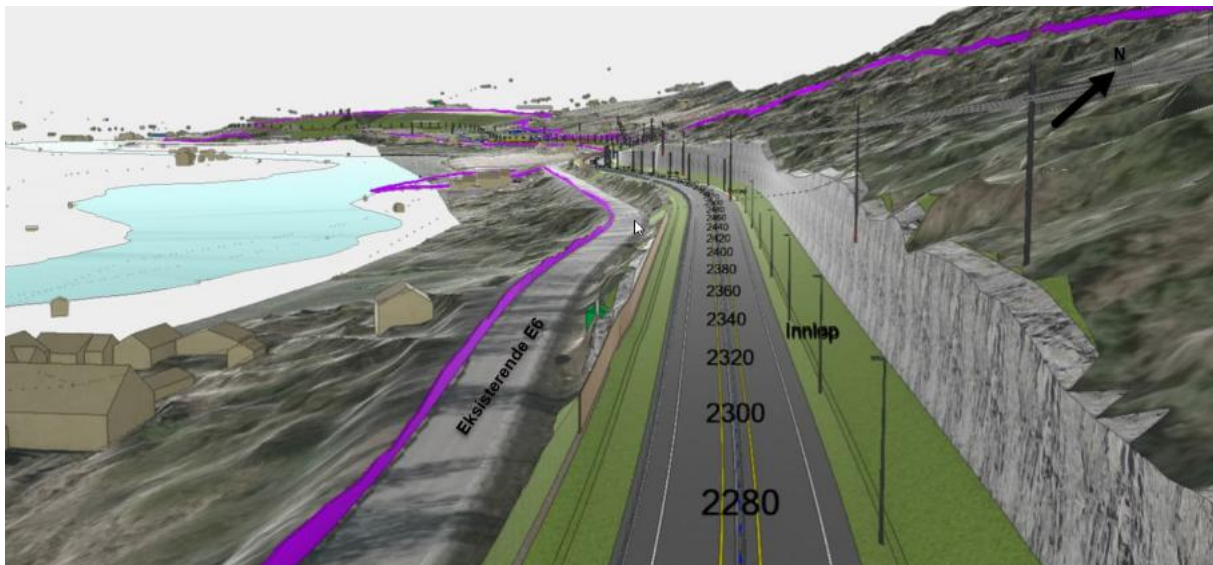
Figur 7-3 Utklipp fra Trimble-modellen. De planlagte bergskjæringene ligger i nærheten til kritisk infrastruktur (E6).
