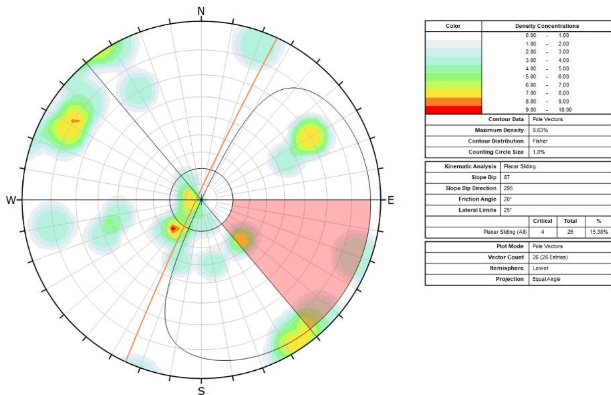
Figur 7: Analyse for planutglidning for skjæring mellom profil 1800-2300.
