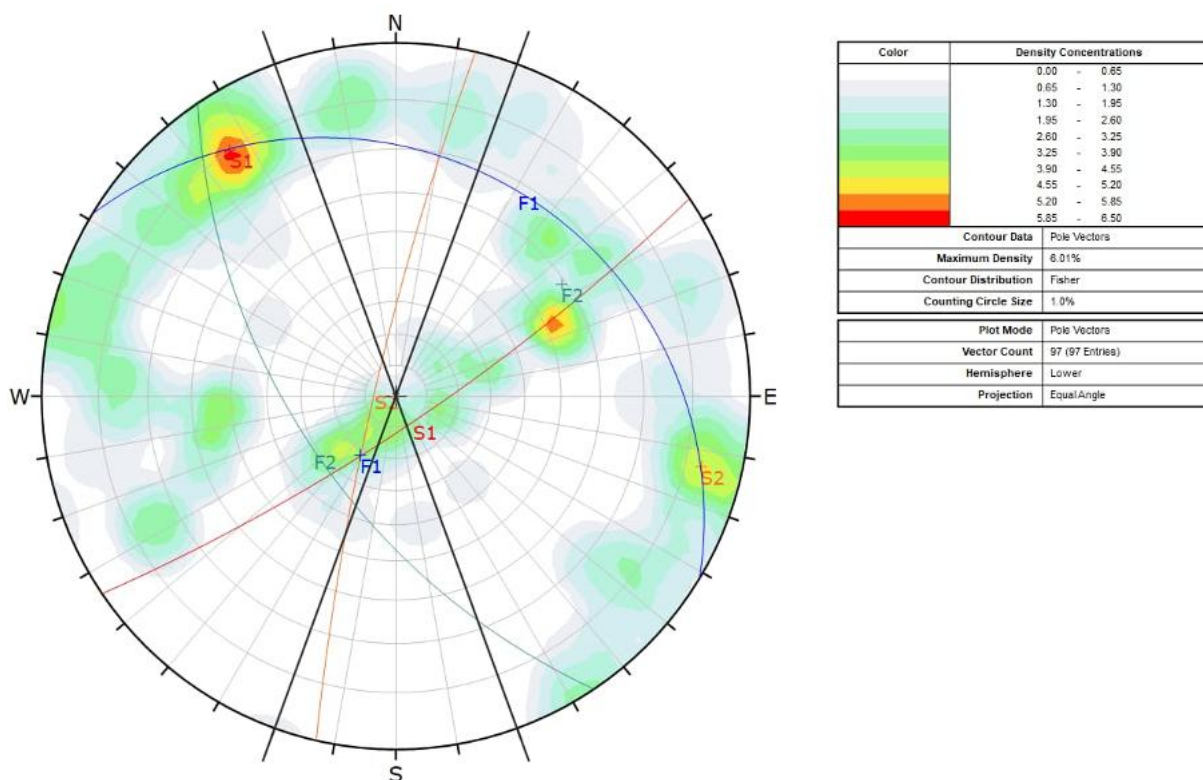
Figur 4-16 Polplott basert på målinger tatt i forbindelse med kartlegging av strekningen Sjoa - Bredevangen.
