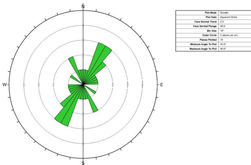
Figur 4-19 Sprekkerose for målinger tatt i forbindelse med kartlegging i området mellom profil 1140-1800. Svart linje indikerer ca. orientering til bergskjæring.
