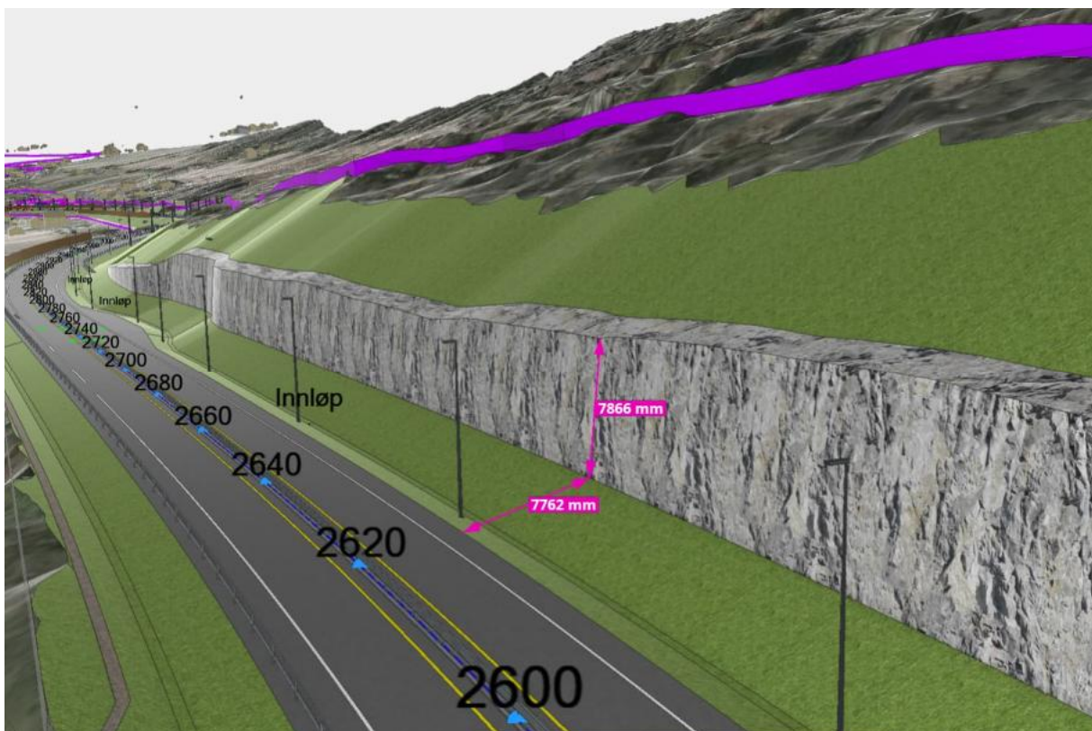
Figur 7-4 Utklipp fra Trimble-modellen. Utklippet viser grøftebredde og skjæringhøyde ved ca. profil 2600.
