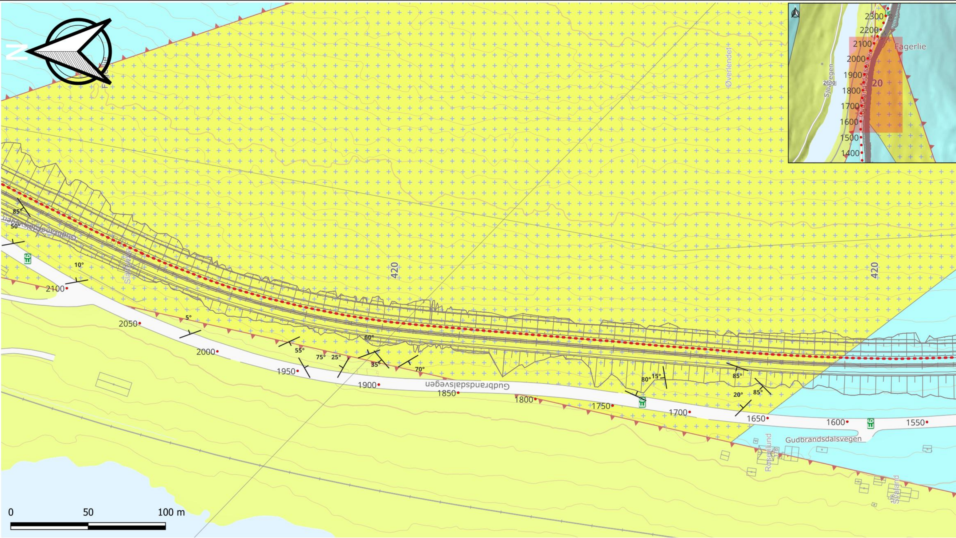
Sprekkeros med målinger fra profil 1600-2300
