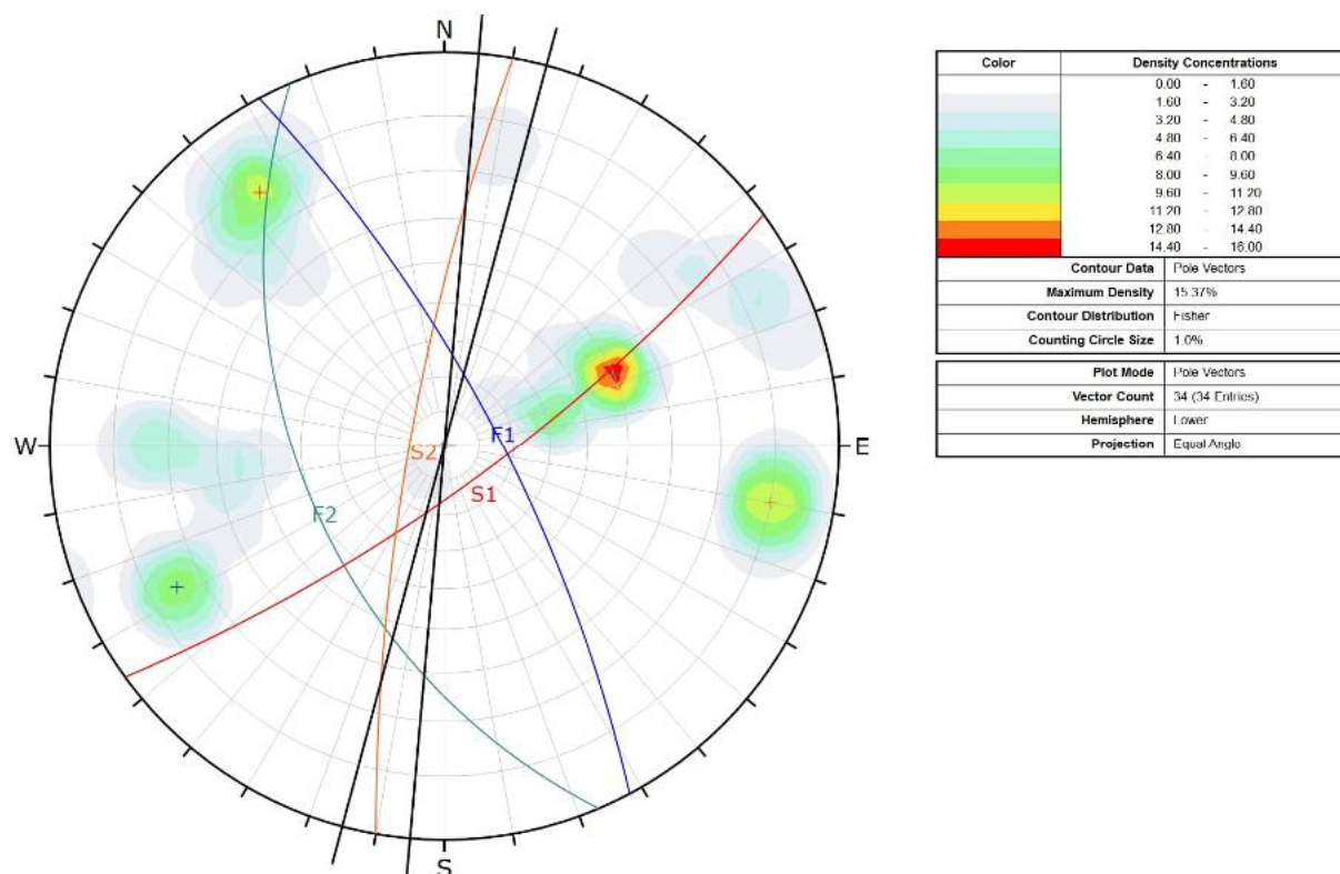
Figur 4-24 Polplott basert på målinger tatt i forbindelse med kartlegging i området mellom profil 2300-2950. Svart linje indikerer ca. variasjon på orientering til bergskjæring.
