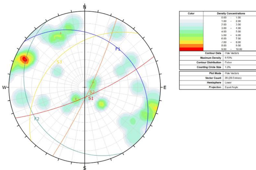
Figur 4-20 Polplott basert på målinger tatt i forbindelse med kartlegging i området mellom profil 1140-1800. Svart linje indikerer ca. orientering til bergskjæring.
