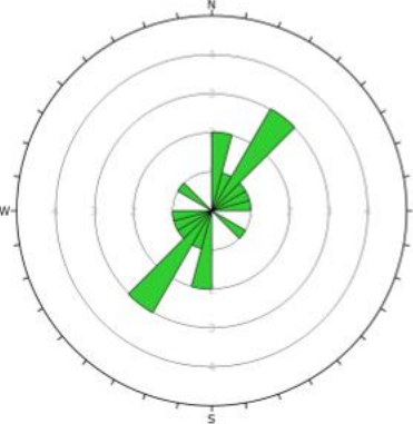
Sprekkeros med målinger fra profil 1000-1400
