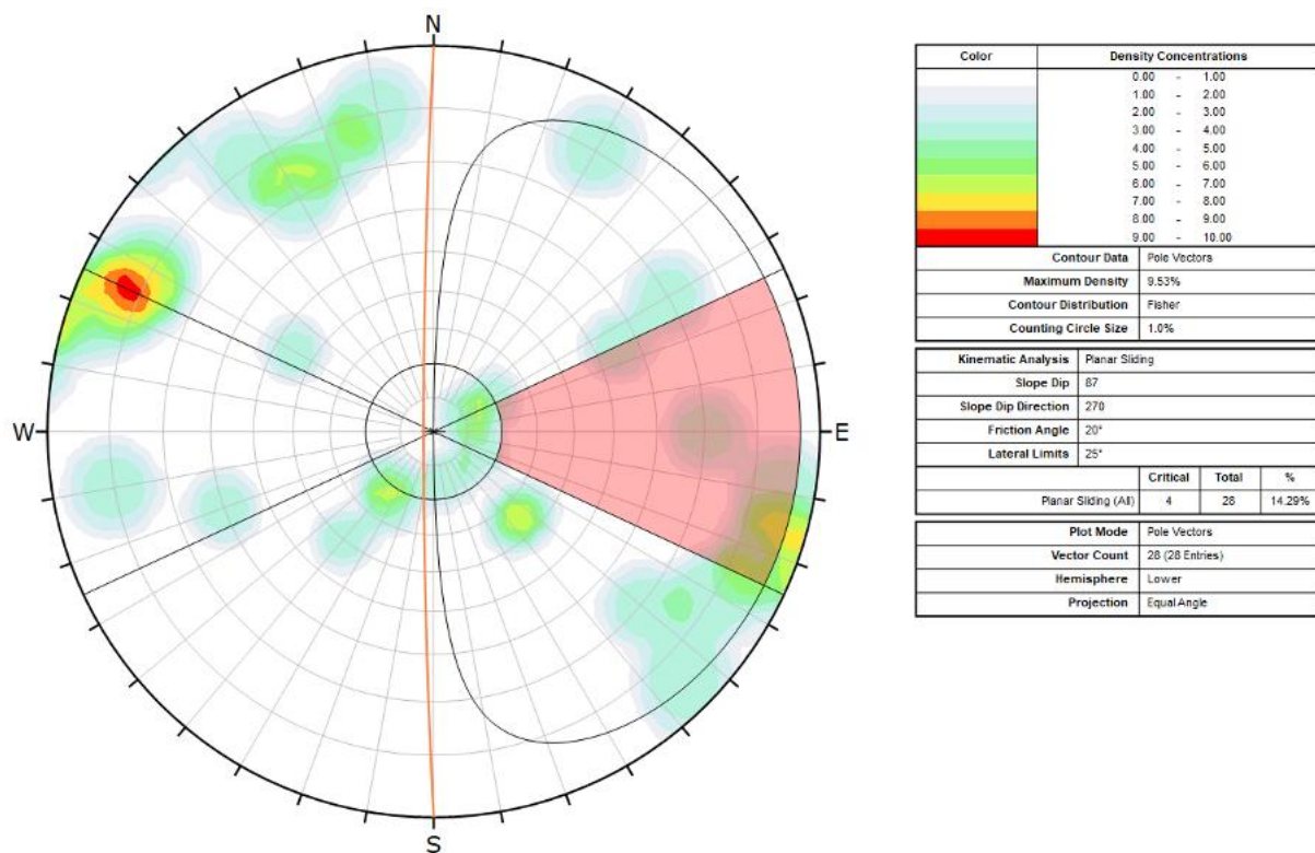
Figur 4: Analyse for planutglidning for skjæring mellom profil 1140-1800
