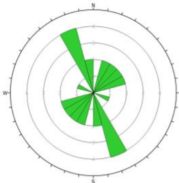
Sprekkeros med målinger fra profil 1600-2300
