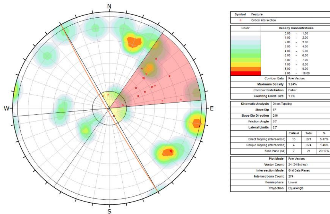
Figur 3: Analyse for toppling/utvelting mellom profil 640-1140
