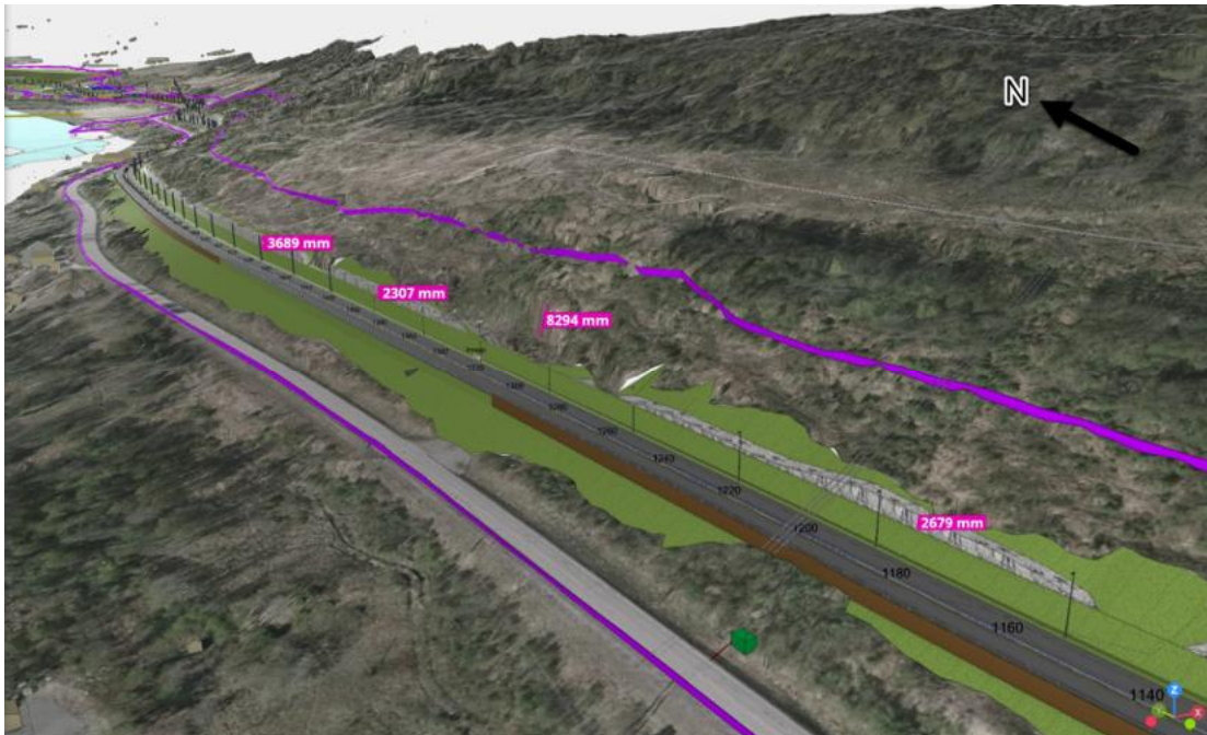
Figur 1-3 Utklipp fra Trimble-modellen. Utklippet viser bergskjæring ved profil 1140-1800. Angitt målt høyde er omtrentlig. Lilla linje er anleggsgrense.
