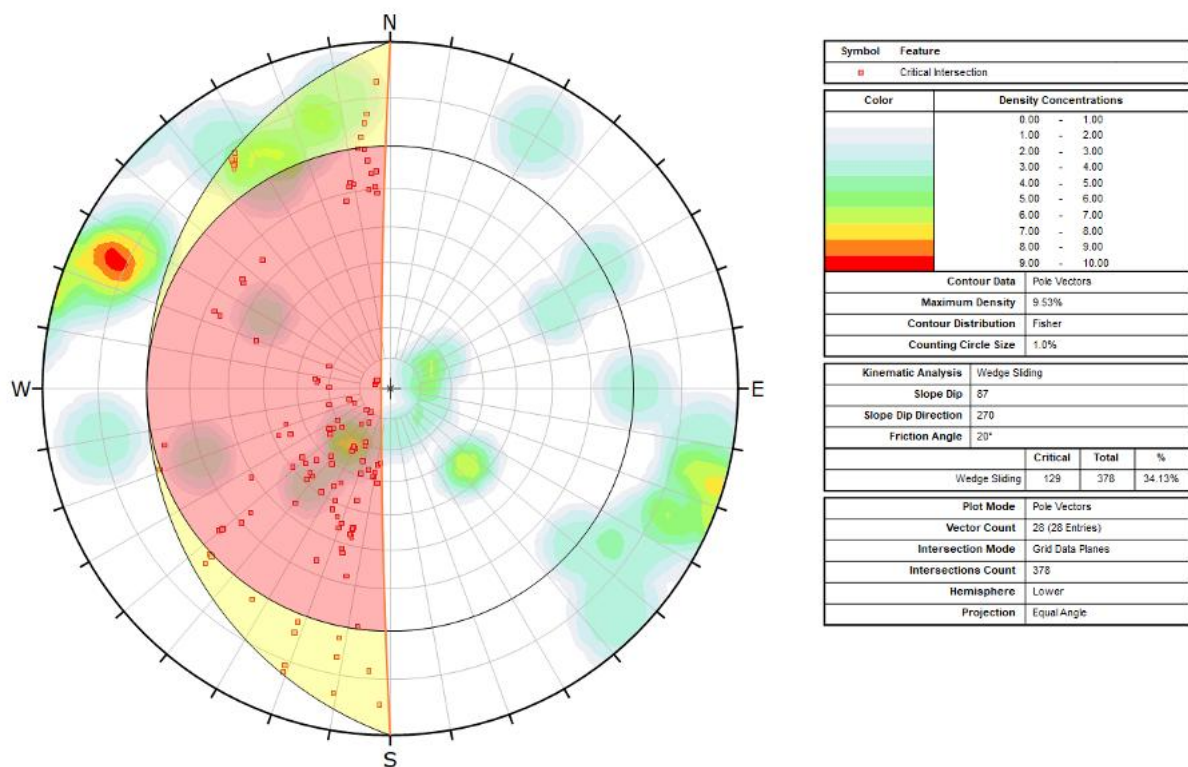
Figur 5: Analyse for kilutglidning mellom profil 1140-1800.
