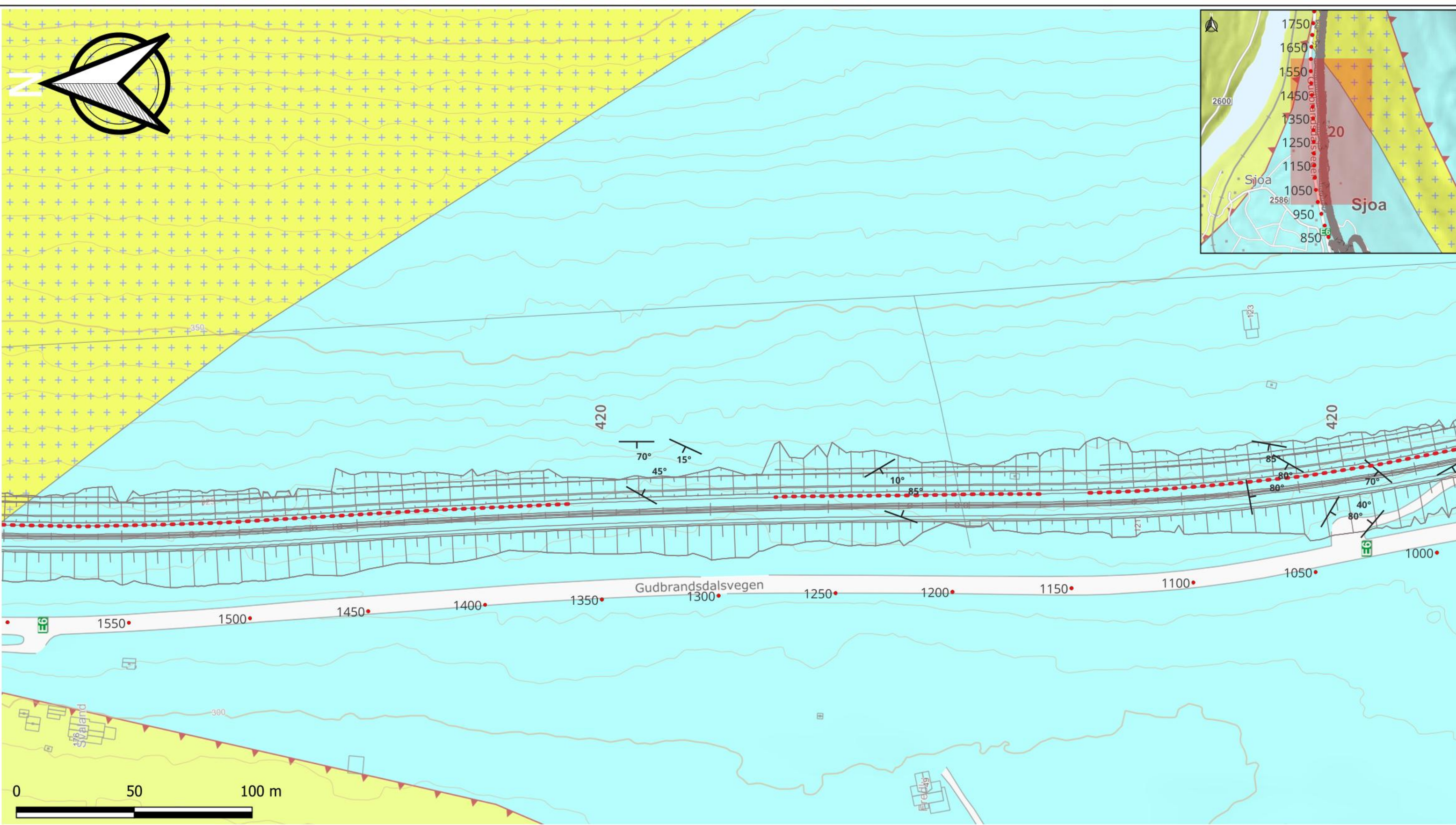
Sprekkeros med målinger fra profil 1000-1400
