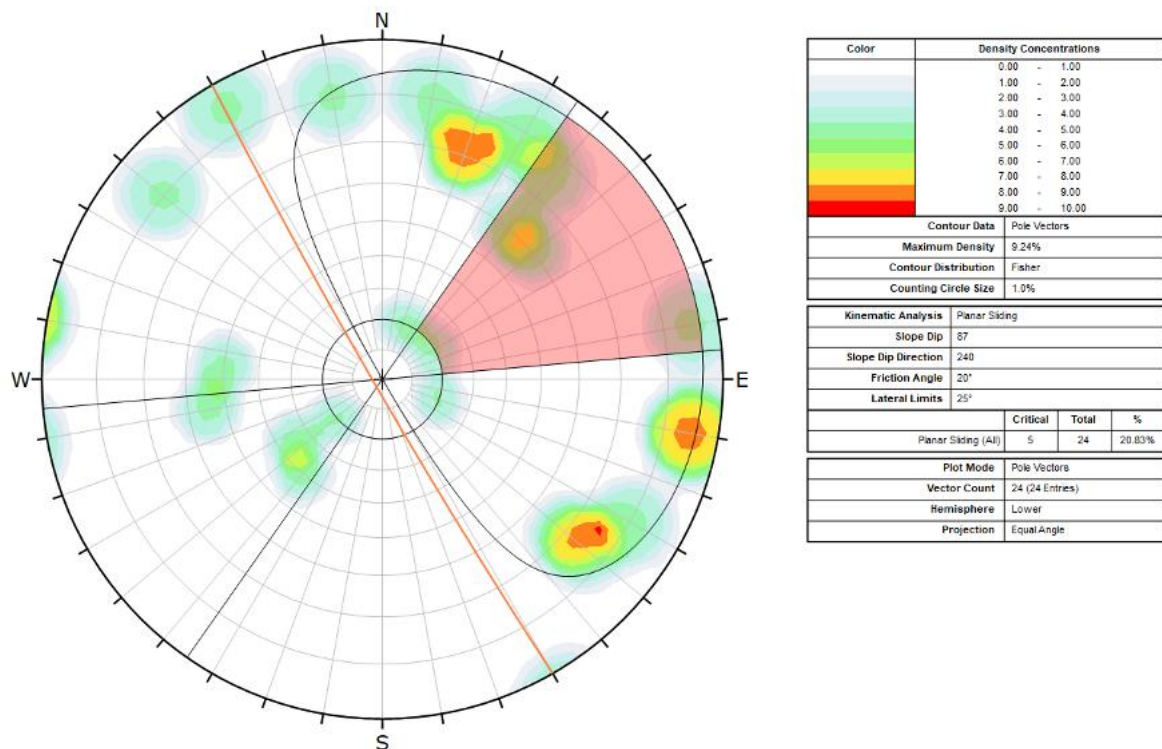
Figure 1: Analyse for planutglidning for skjæring mellom profil 640-1140
