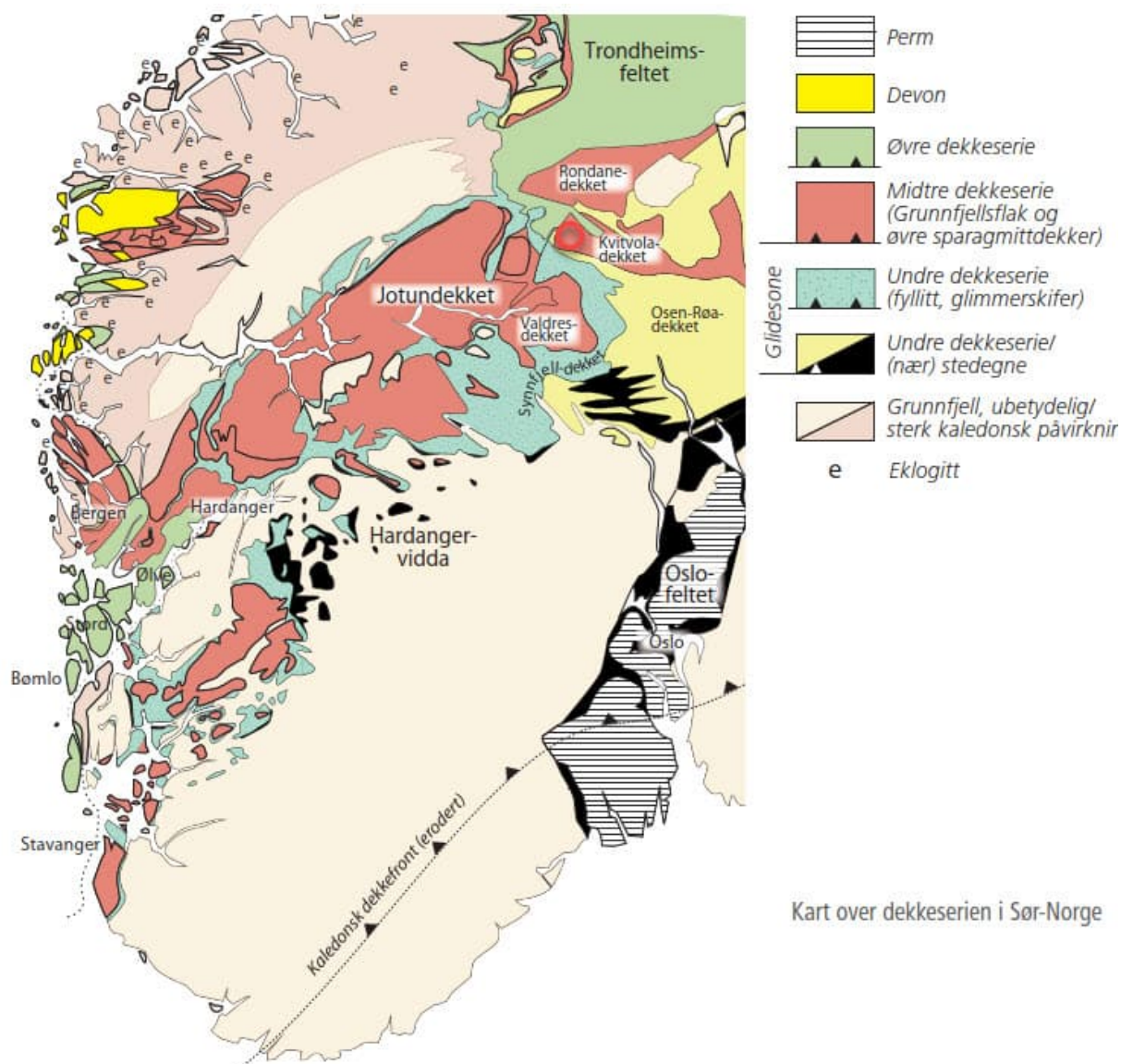
Figur 4-3 Kart over dekkeserien i Sør-Norge hentet fra [18]. Området Sjøa - Bredevangen er omtrentlig markert med rød sirkel.
