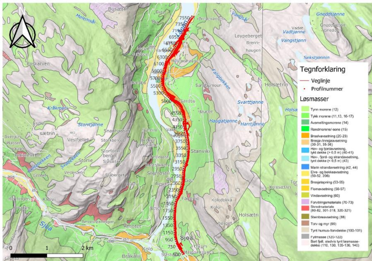
Figur 5-2 Løsmassekart med grunnlag fra NGU.
