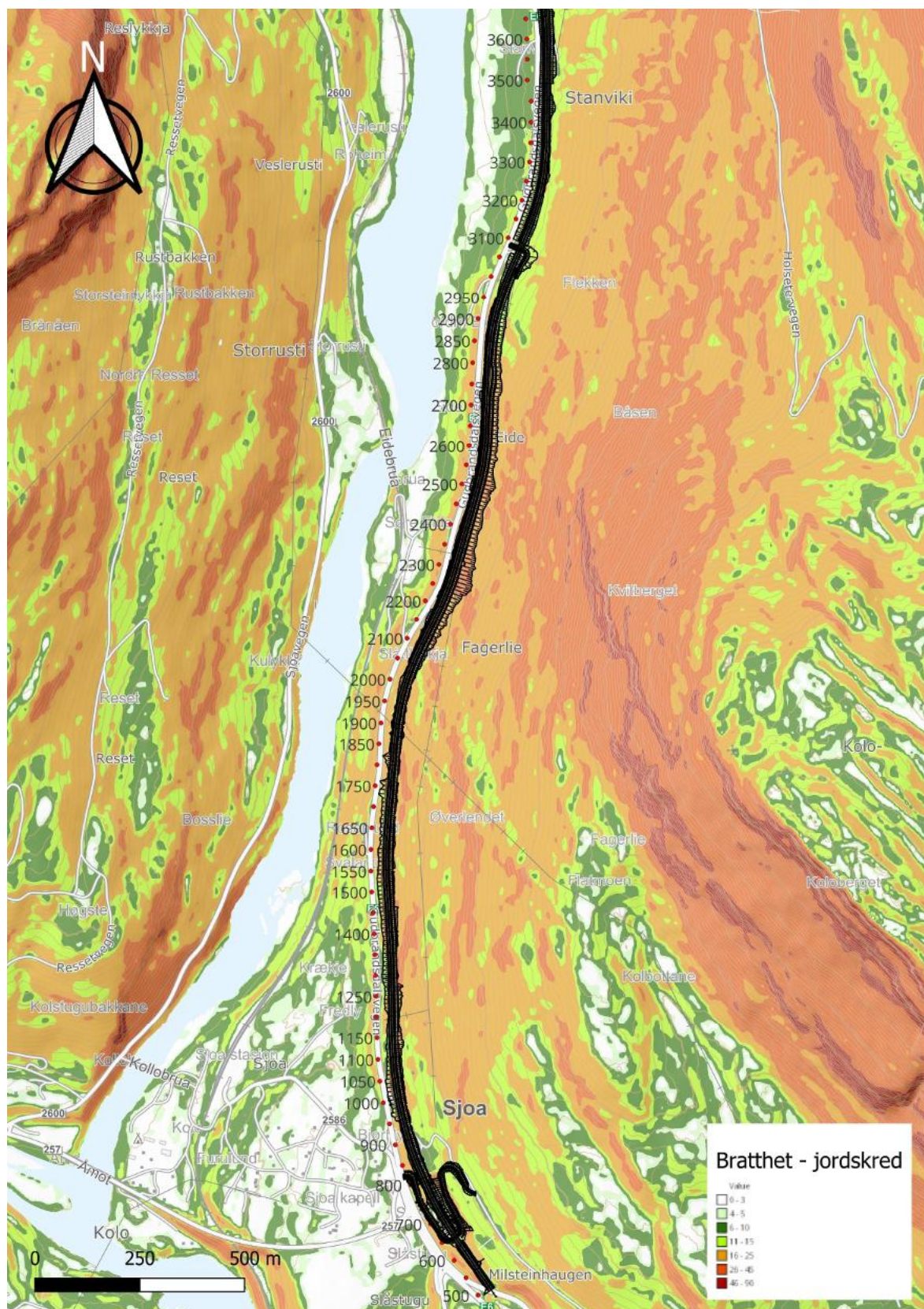
Figur 5-1 Bratthetskart. WMS-kart hentet fra Geonorge og grunnlag fra NVE.
