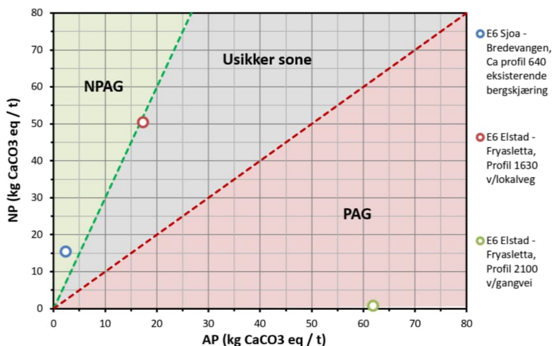
Figur 3-1 Fra /16/. Vurdering av total syredanningspotensiale basert på beregning av Neutralization Potential Ratio ( NPR = NP/AP , med NP: nøytraliseringspotensial og AP: Syredanningspotensial). NPAG: Non Potentially Acid Generating; PAG: Potentially Acid Generating. Merk at prøvene fra E6 Elstad – Fryasletta ikke er relevant for denne rapporten.
