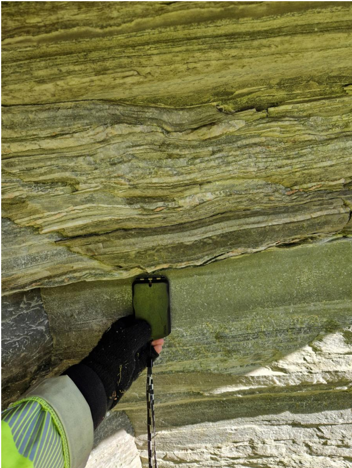
Figur 4-13 Vekslende lag av dolomittmarmor og sandstein med karbonatlag.
