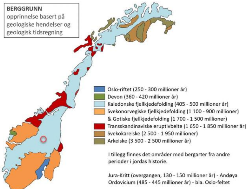
Figur 4-1 Geologiske hendelser i Norge fra geogleblog.com. Området Sjøa - Bredevangen er omtrentlig markert med rød sirkel.
