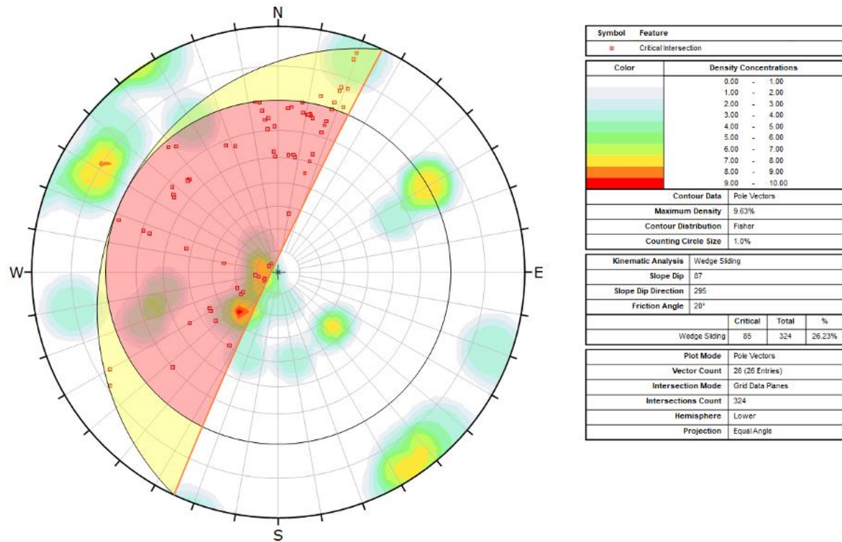
Figur 8: Analyse for kilutglidning mellom profil 1800-2300.
