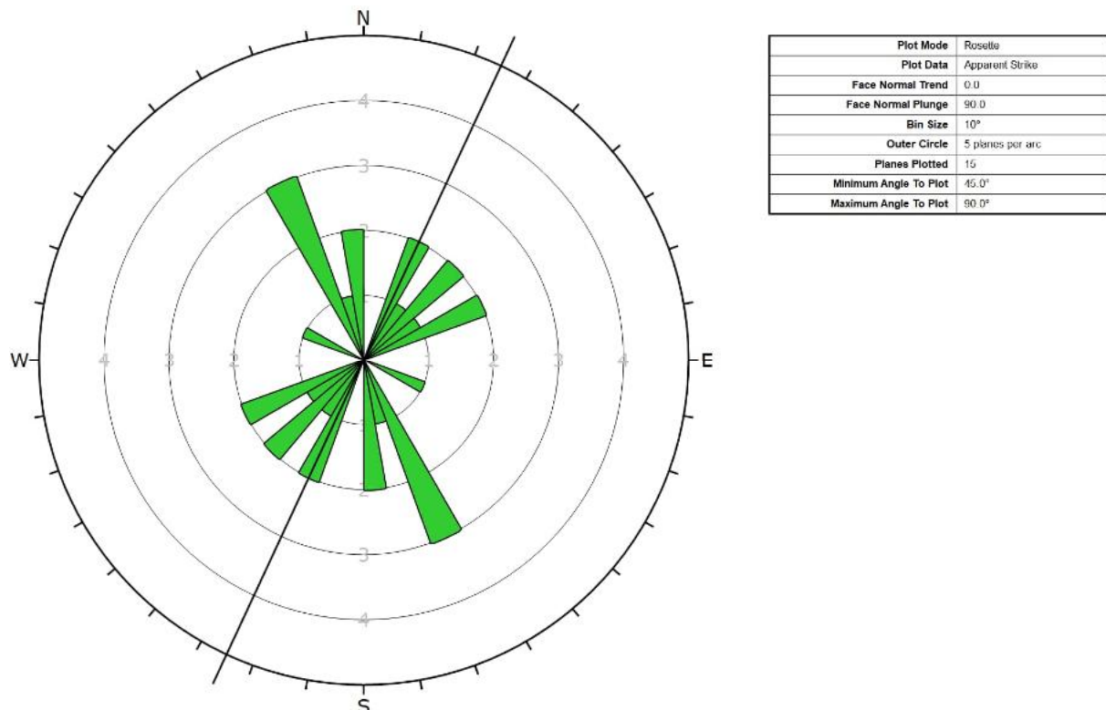
Figur 4-21 Sprekkerose for målinger tatt i forbindelse med kartlegging i området mellom profil 1800-2300. Svart linje indikerer ca. orientering til bergskjæring.
