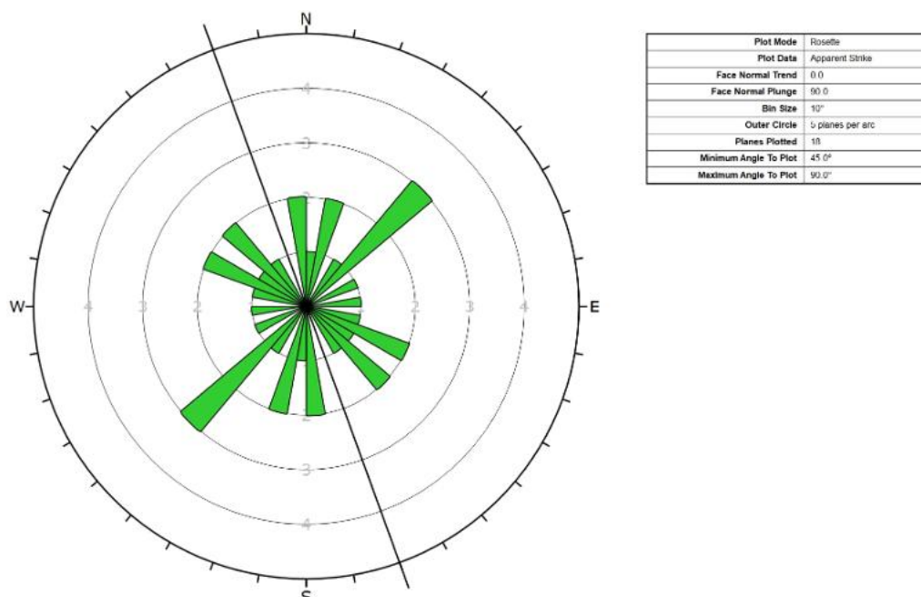
Figur 4-17 Sprekkerose for målinger tatt i forbindelse med kartlegging i området mellom profil 640-1140. Svart linje indikerer ca. orientering til bergskjæring.
