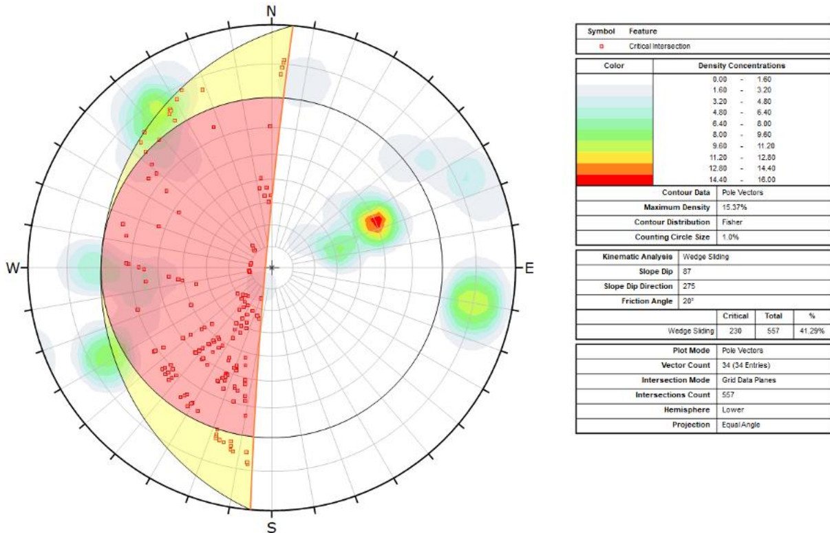
Figur 11: Analyse for kilutglidning mellom profil 2300-2900.
