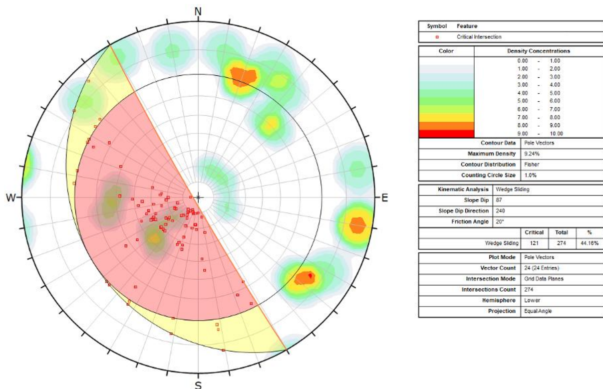
Figure 2: Analyse for kilutglidning mellom profil 640-1140
