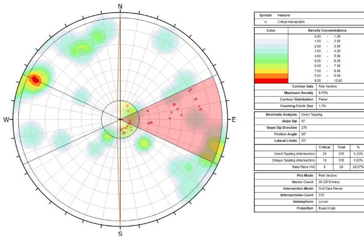
Figur 6: Analyse for toppling/utvelting mellom profil 1140-1800
