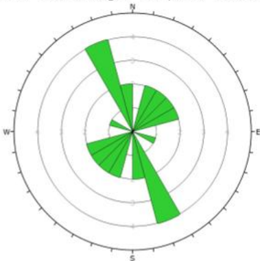
Sprekkeros med målinger fra profil 1600-2300
