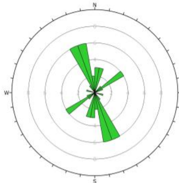
Sprekkeros med målinger fra profil 2300-2900
