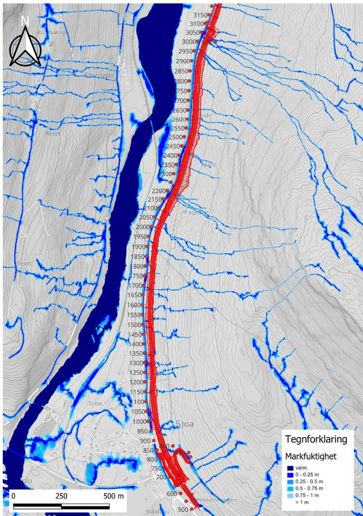
Figur 5-4: Markfuktighetskart fra NIBIO
