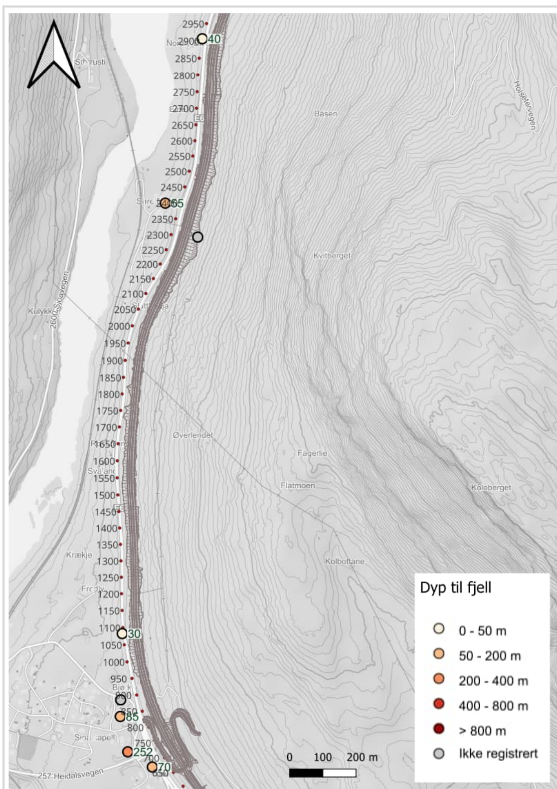
Figur 5-5: Registrerte brønner i GRANADA langs strekning med bergskjæring.
