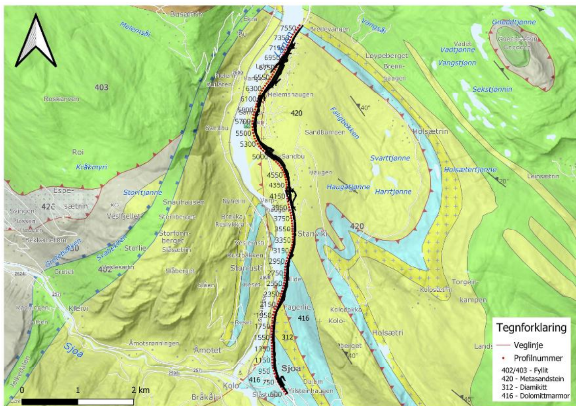
Figur 4-2 Oversikt av regional berggrunnskart 1:250 000 oversiktskart med veglinje og profilnummer. WMS-kartet er hentet fra GeoNorge med grunnlag fra NGU.
