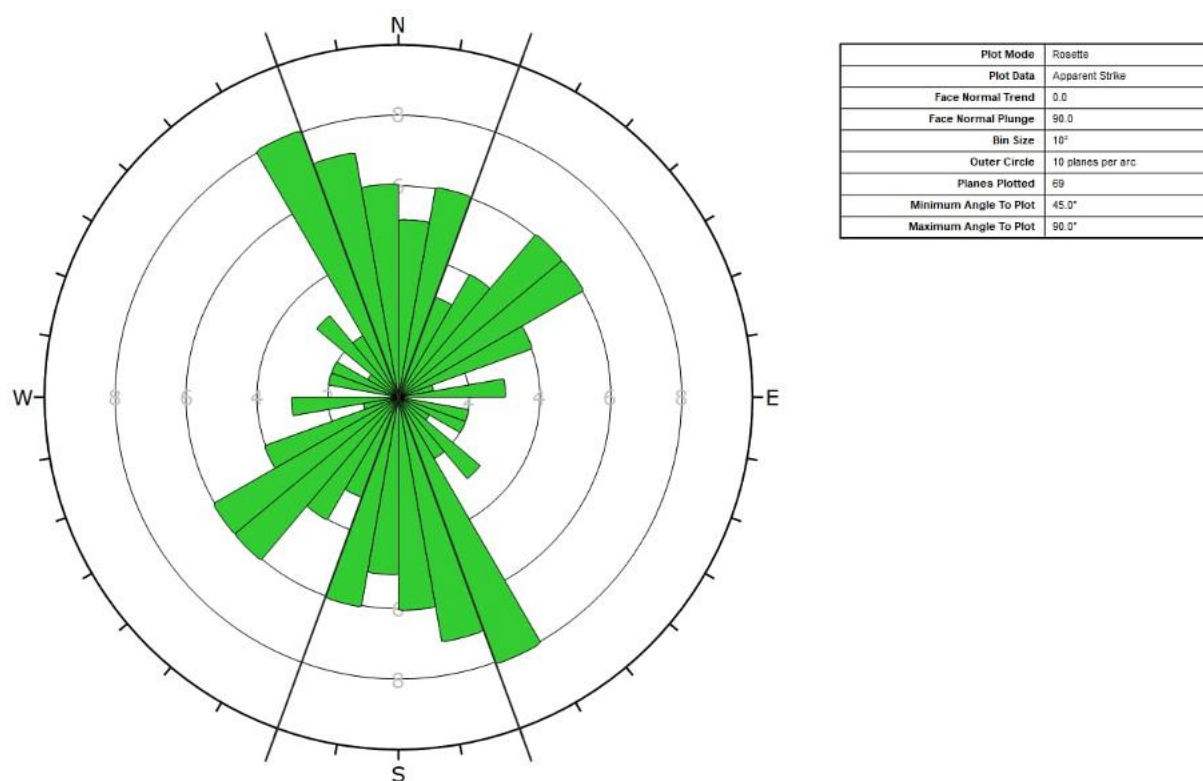
Figur 4-15 Sprekkerose for målinger tatt i forbindelse med kartlegging i området Sjoa - Bredevangen.
