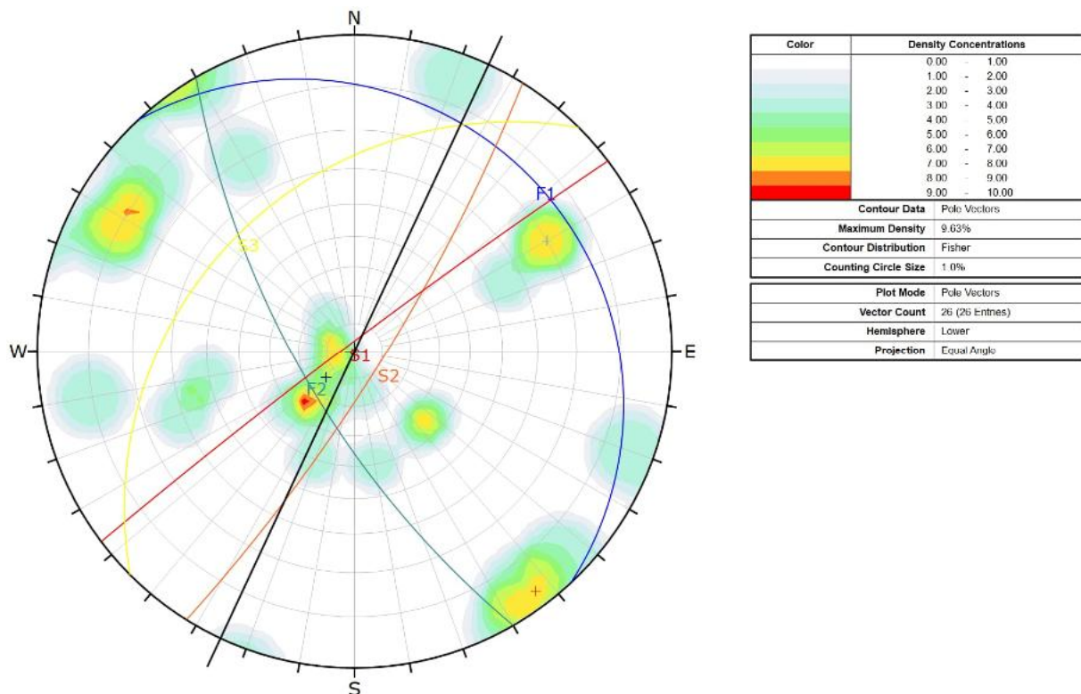
Figur 4-22 Polplott basert på målinger tatt i forbindelse med kartlegging i området mellom profil 1800-2300. Svart linje indikerer ca. orientering til bergskjæring.
