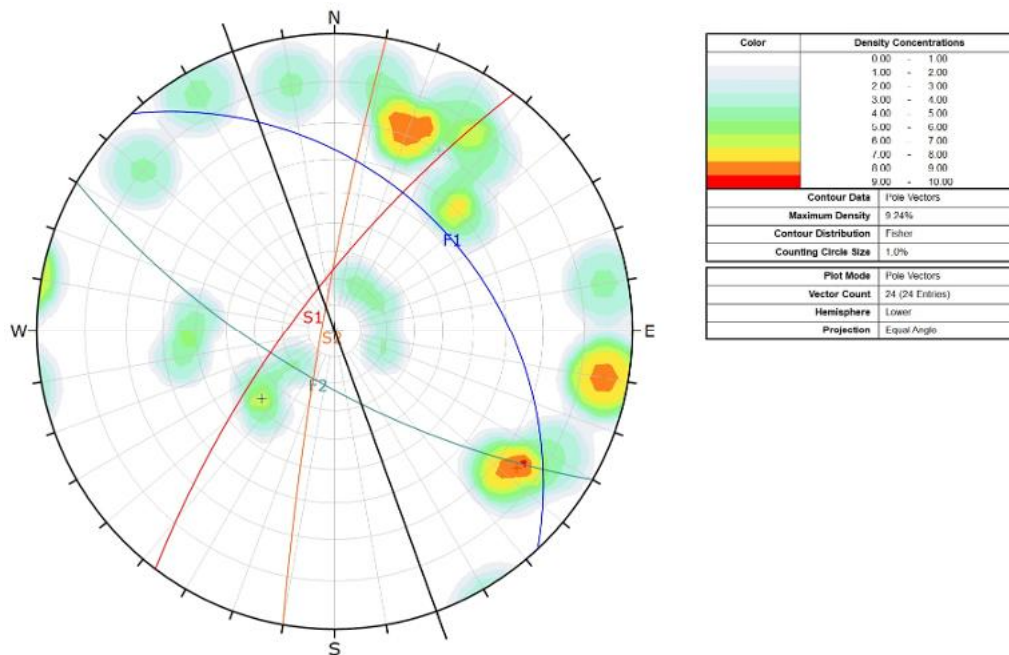
Figur 4-18 Polplott basert på målinger tatt i forbindelse med kartlegging i området mellom profil 640-1140. Svart linje indikerer ca. orientering til bergskjæring.
