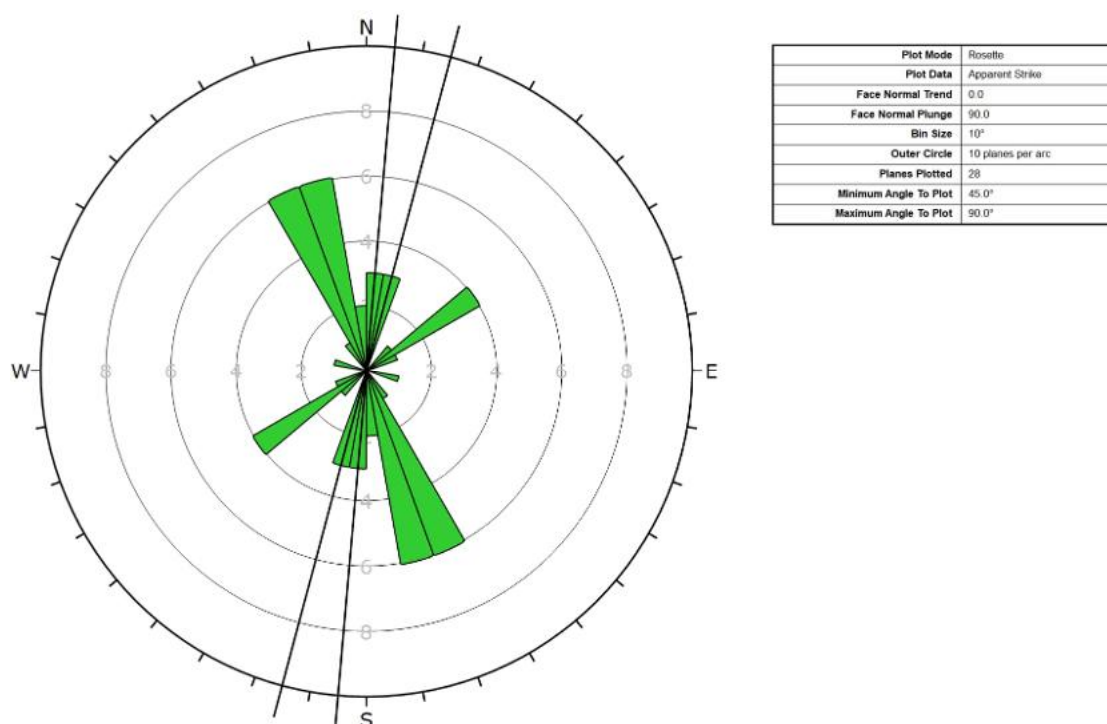
Figur 4-23 Sprekkerose for målinger tatt i forbindelse med kartlegging i området mellom profil 2300-2950. Svart linje indikerer ca. variasjon på orientering til bergskjæring.
