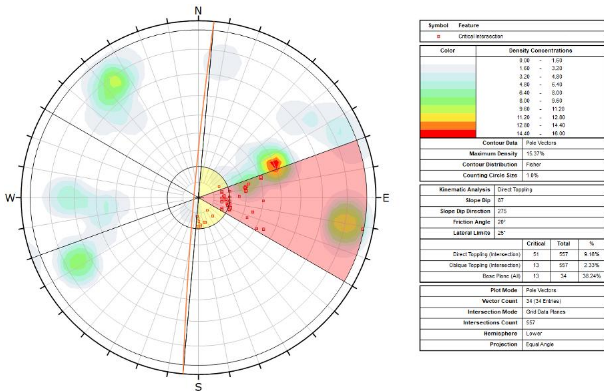
Figur 12: Analyse for toppling/utvelting mellom profil 2300-2900.
