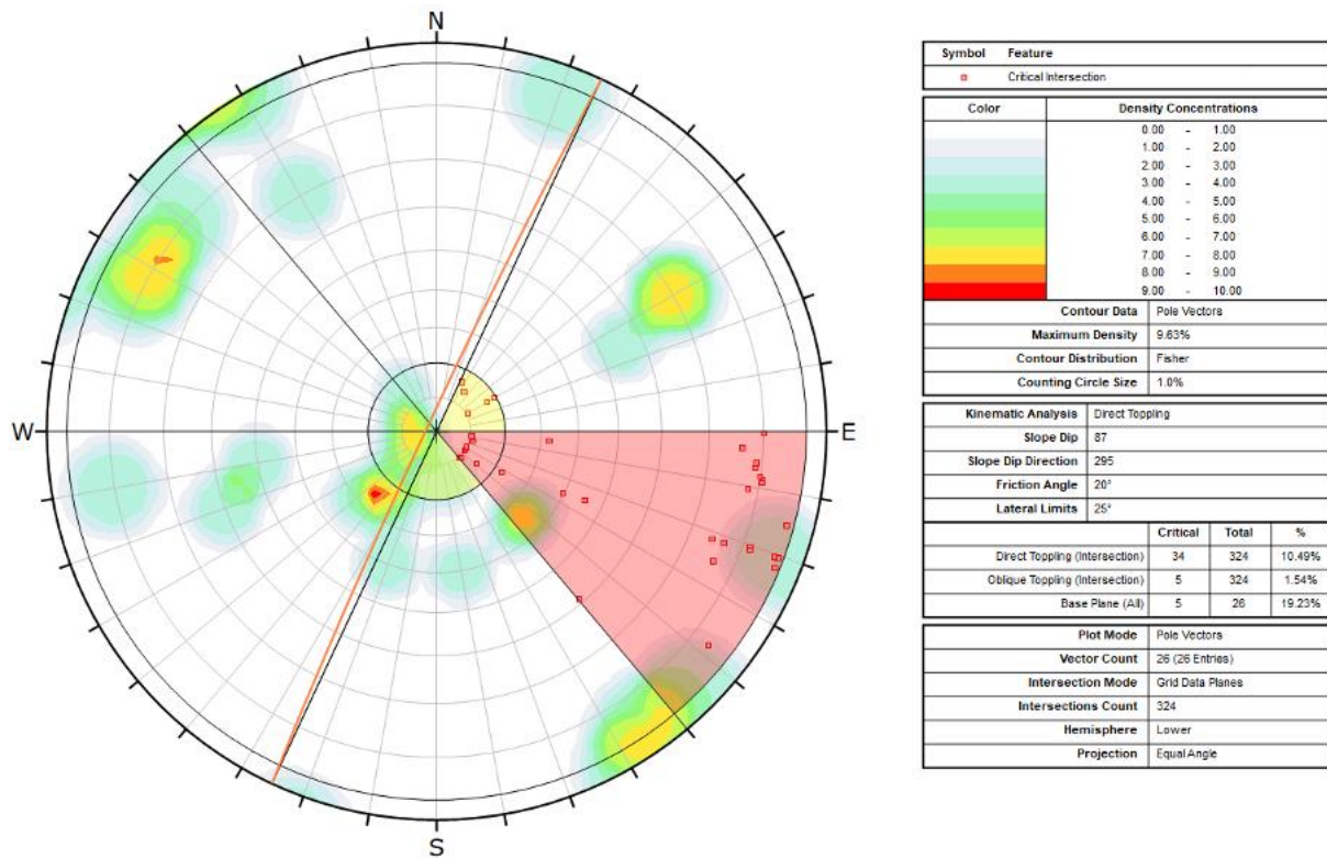
Figur 9: Analyse for toppling/utvelting mellom profil 1800-2300.
