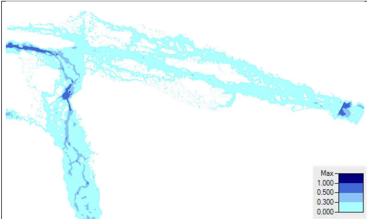
Figur 11: Vandedybde [m] i bekkene på Mysusæter, 200-årsflom inkl. 40% klimapåslag.
