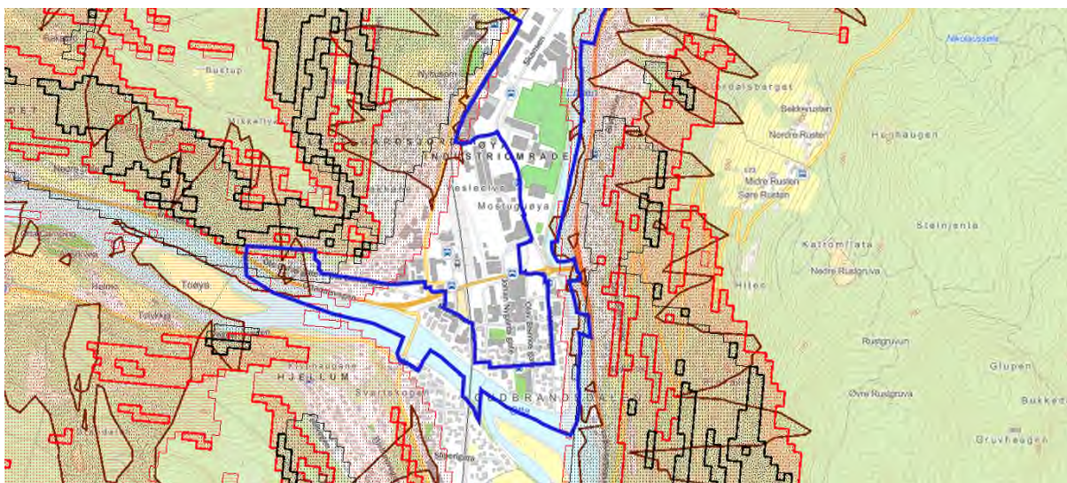
Figur 12. Kartutsnittet viser aktsomhet skred for søre del av planområdet. Svart angir steinsprang, rødt snøskred og brunt jord- og flomskred. Blå strek angir plangrense. Kilde kartgrunnlag: InnlandsGIS
