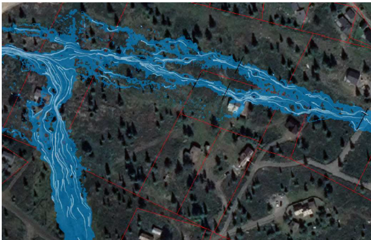
Figur 10. Flomutbredelse med strømlinjer (hvite linjer) angitt for 200-års flom med 40% klimapåslag. Kilde: Flomutredning Mysusæter, Norconsult 15.07.21
