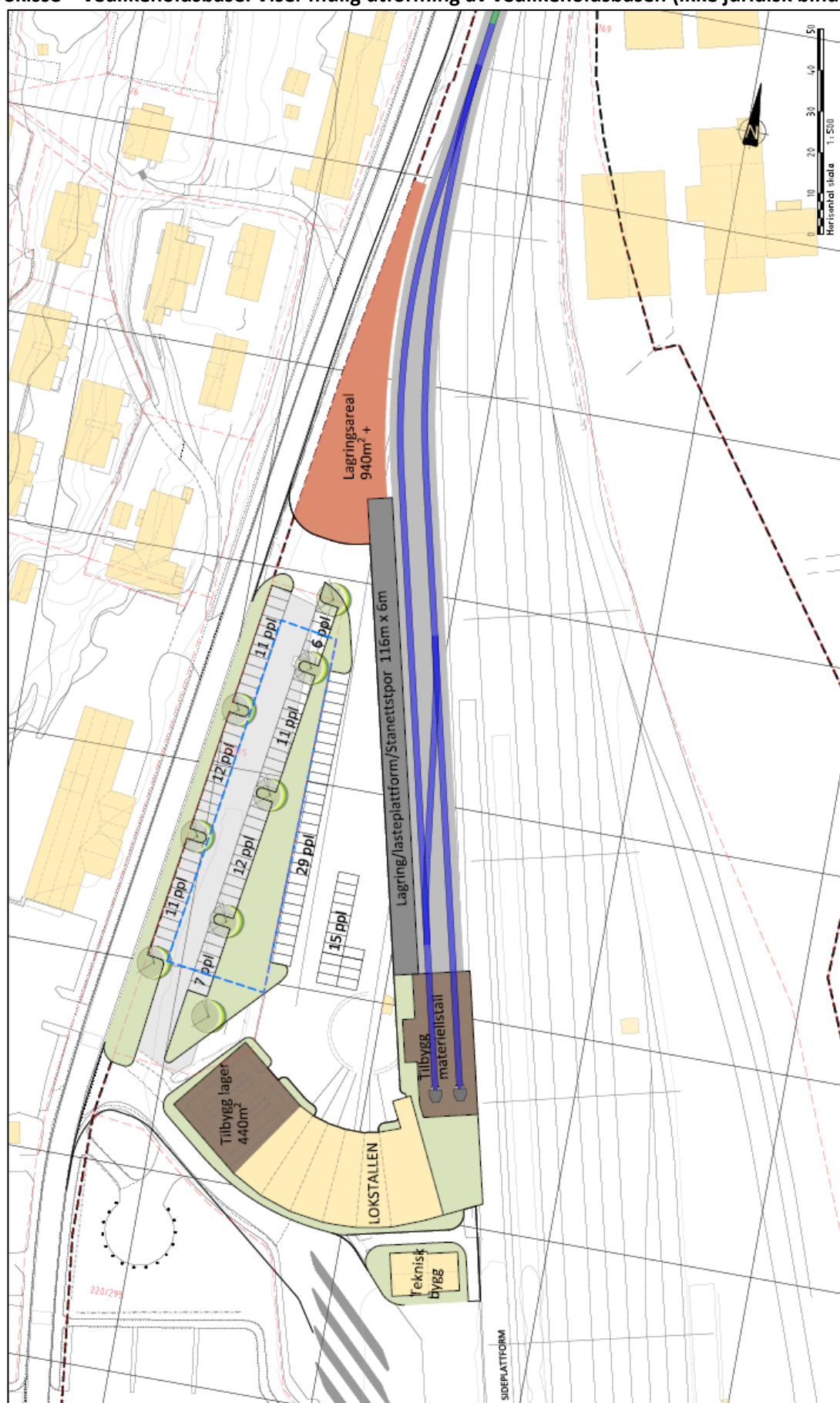
Skisse – vedlikeholdsbase. Viser mulig utforming av vedlikeholdsbasen (ikke juridisk bindende)
