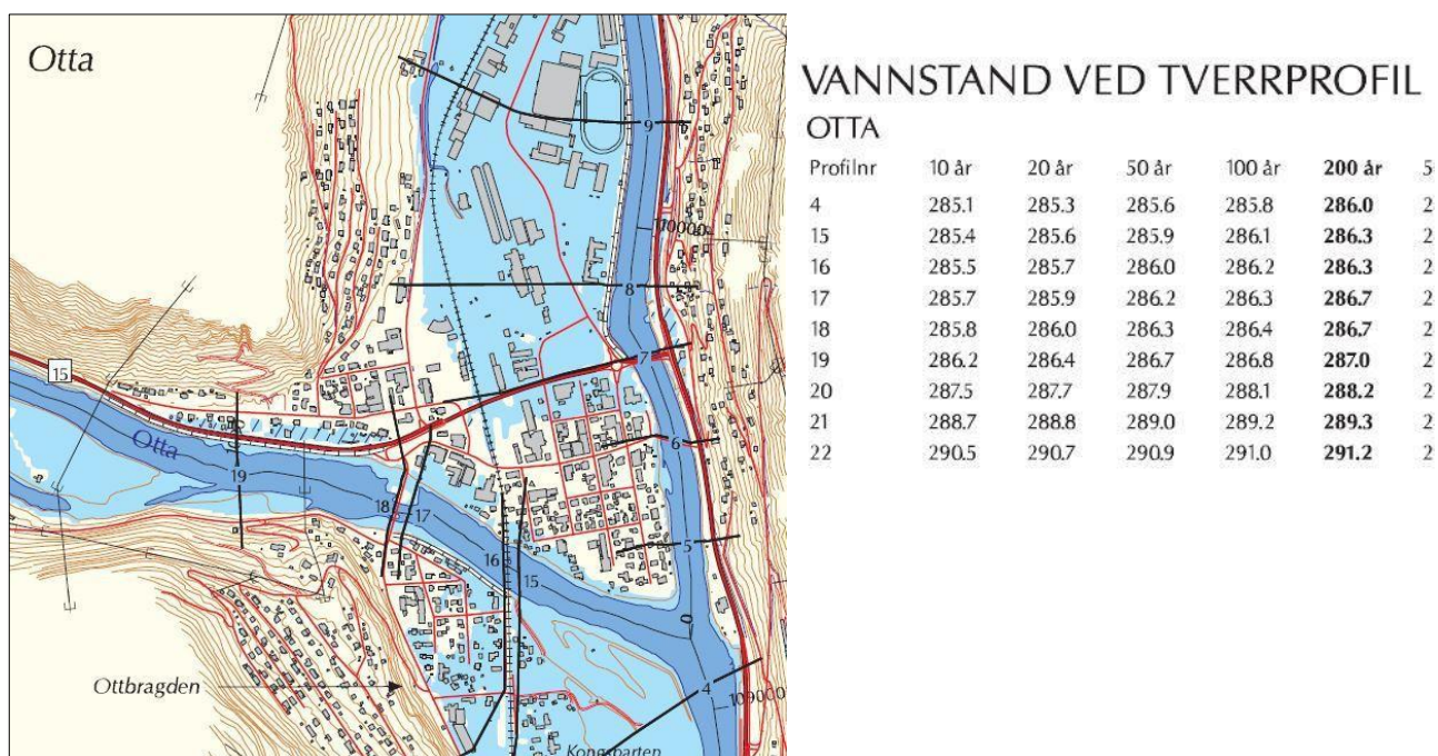
Figur 5-10: Flomsonekart for Otta viser 200-års-flom. Kilde: NVE
