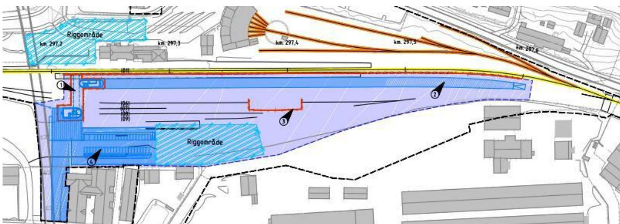
Figur 9-2: Fase 00.40 bygging av ny mellomplattform og ferdigstillelse av kulvert del 1
