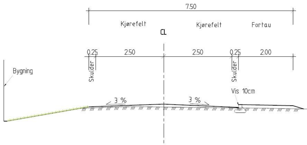
Figur 7-2 Normalprofil for veg til bussterminal
