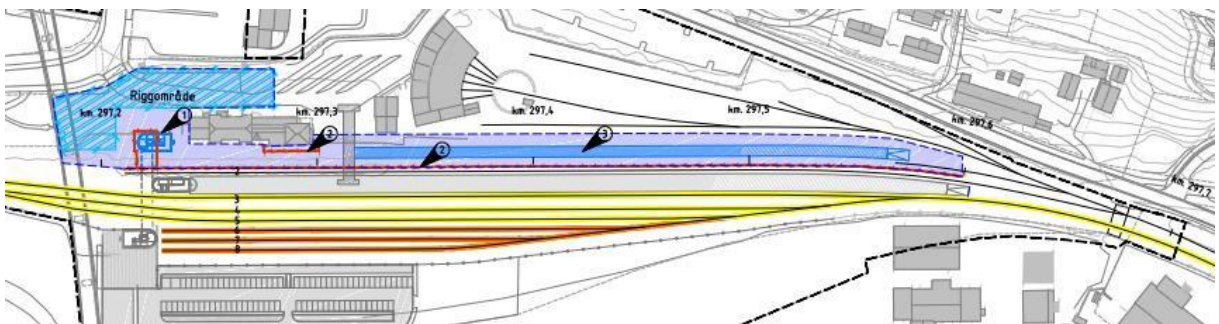
Figur 9-4: Fase 10.30 bygging av ny sideplattform og ferdigstillelse av undergang
