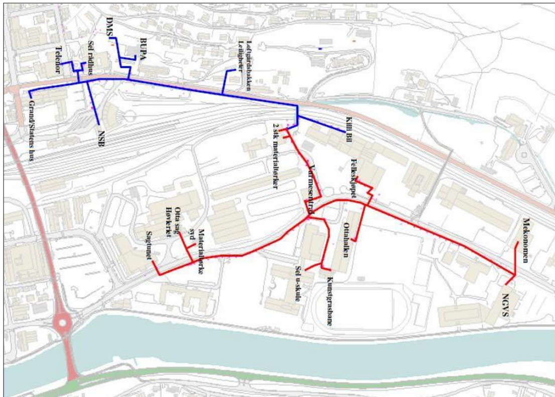
Figur 5-7 Otta fjernvarmes anlegg ved planområdet
