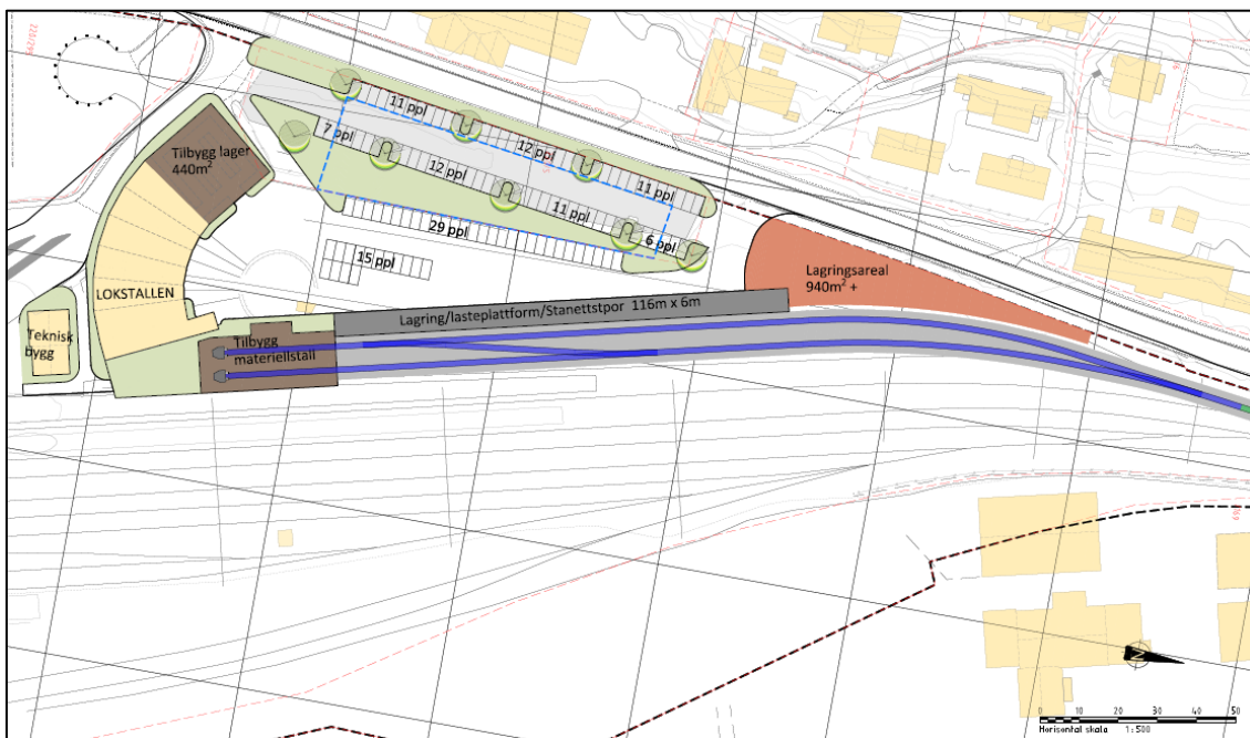
Figur 6-1 Mulig disponering av arealene ved utvidelse av vedlikeholdsbase/ lokstall
